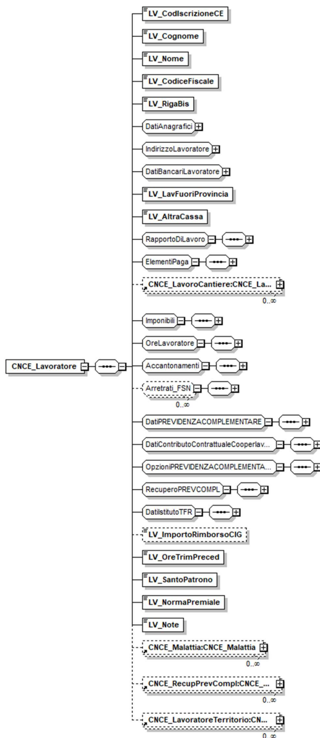
Figura 5: struttura Lavoratore
