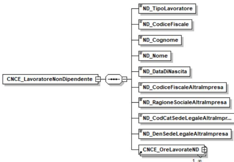
Figura 9: struttura LavoratoreNonDipendente
