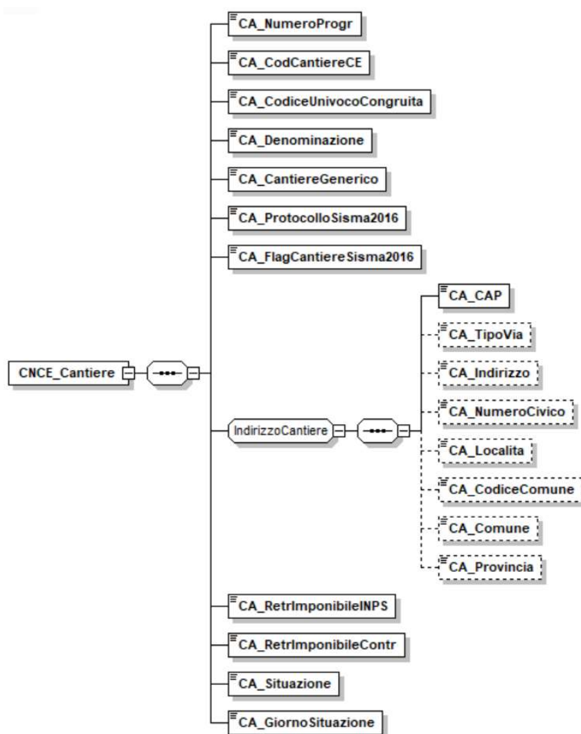
Figura 4: struttura Cantiere
