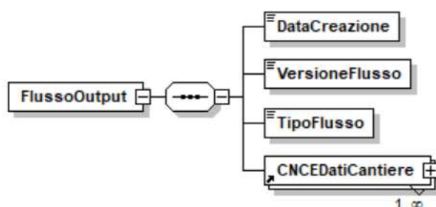
Figura 12: Struttura FlussoOutput
