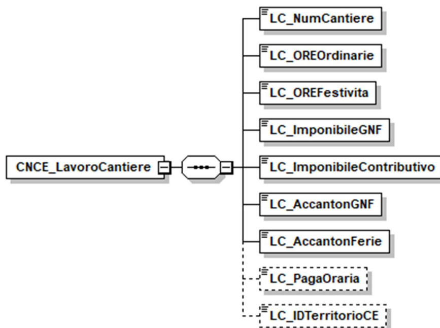
Figura 6: struttura LavoroCantiere
