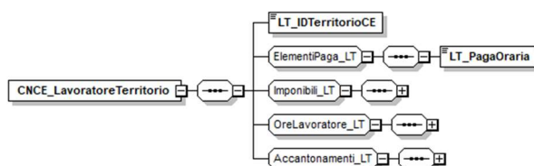
Figura 15: struttura LavoratoreTerritorio
