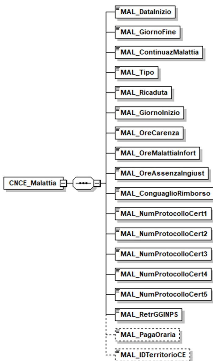
Figura 7: struttura Malattia
